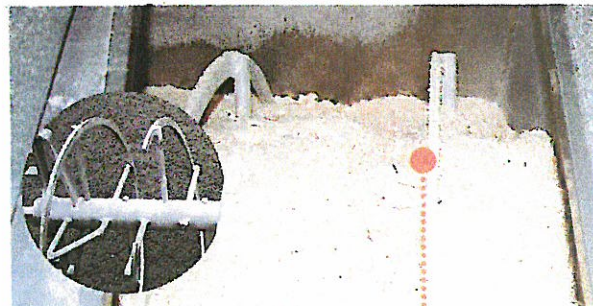
強化スクリューには数々の特許が使われています。圧力に耐える工夫と隅部の攪拌、全体の攪拌効率とデットスペースの解消等の特長を有しています。
